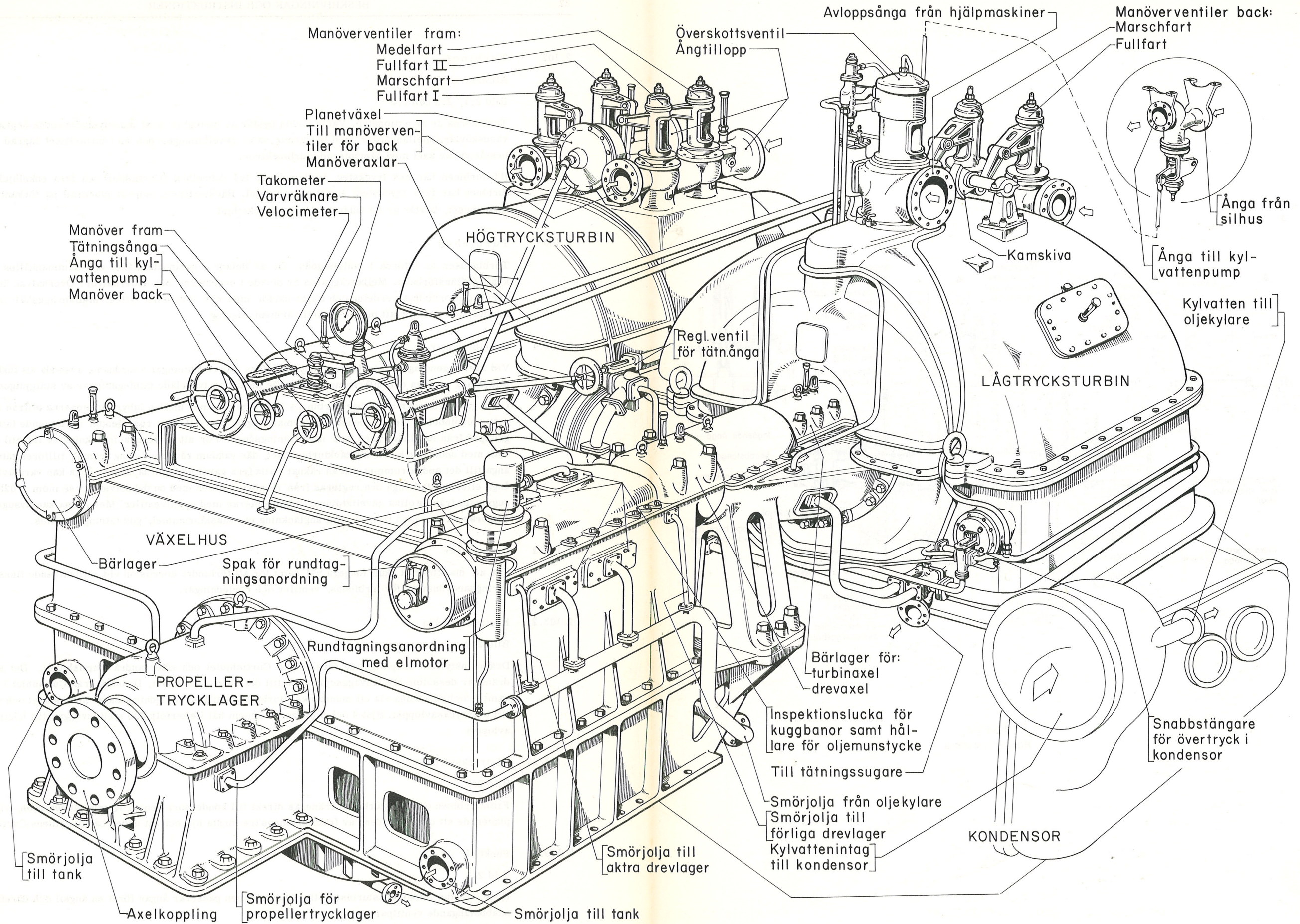
Bild 2:1 Huvudmaskineri Sammanställning
